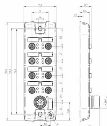
ASBSV-R/ASBSV-R... LED
