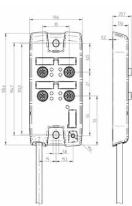
ASB-R/ASB-R... LED
